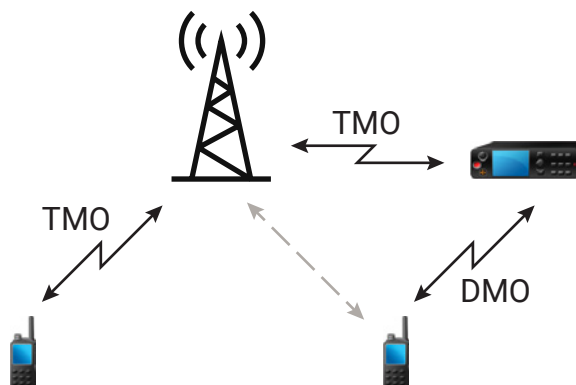
Abbildung 7: Kommunikation über Gateways
