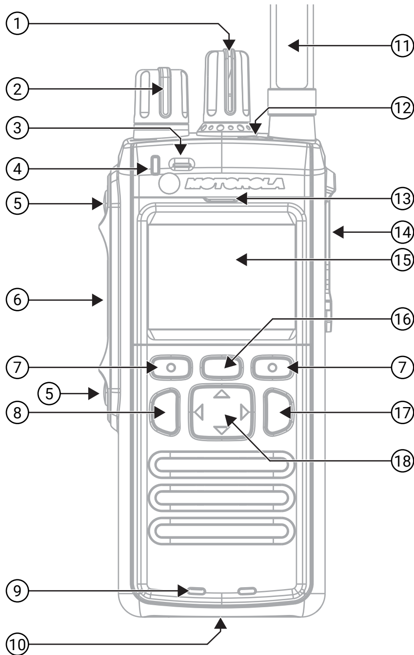
Abbildung 2: Bedienelemente und Anzeigen der Serie MTP3x00
