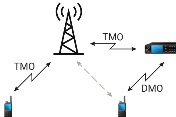
Abbildung 6: Kommunikation über Gateways
