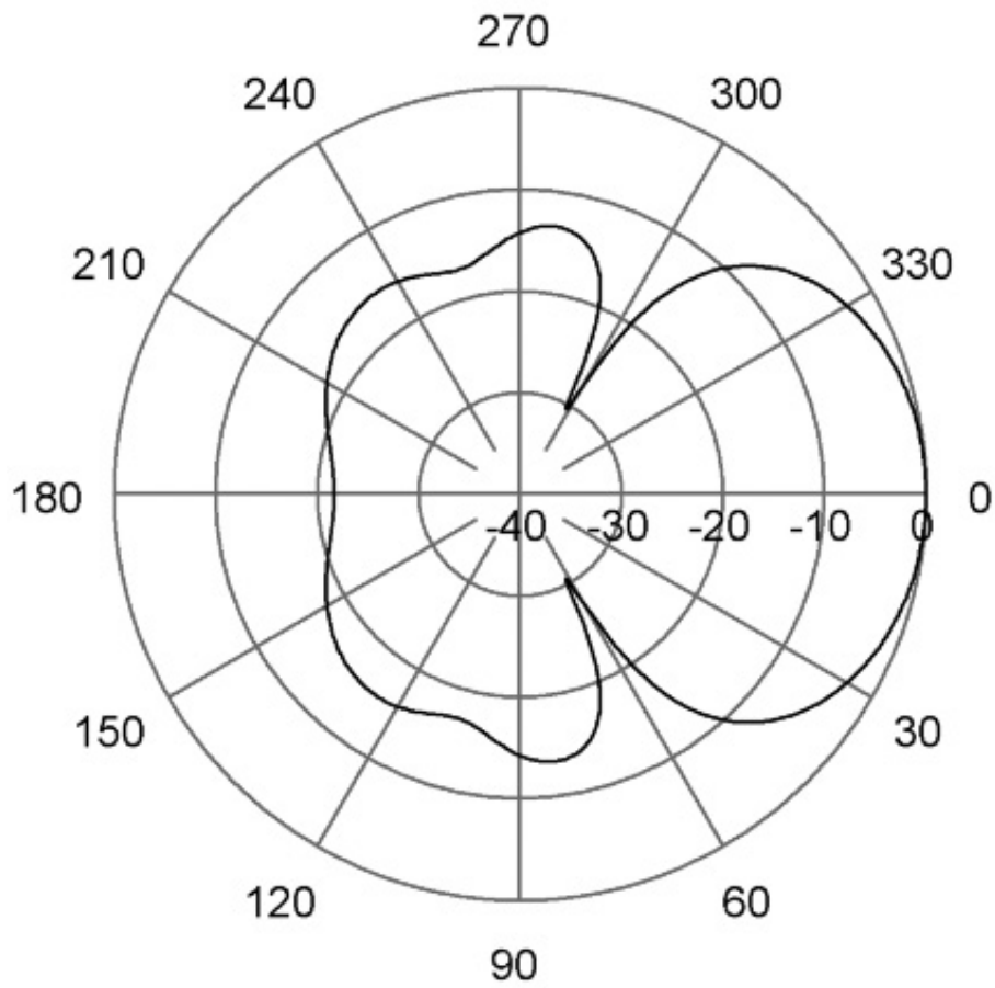
H-Plane | 165 MHz
