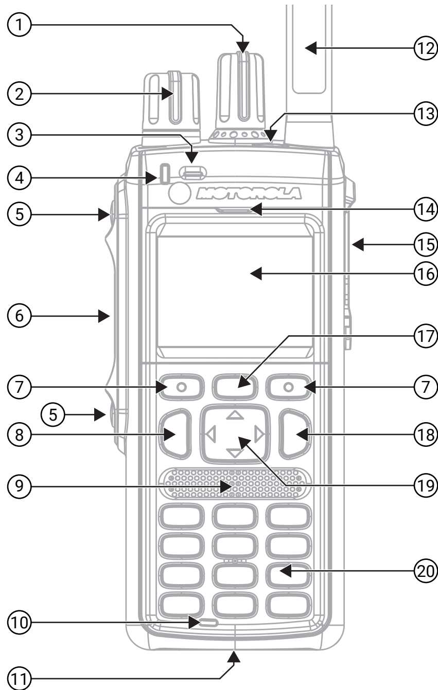
Abbildung 2: Bedienelemente und Anzeigen der Serie MTP3x50
